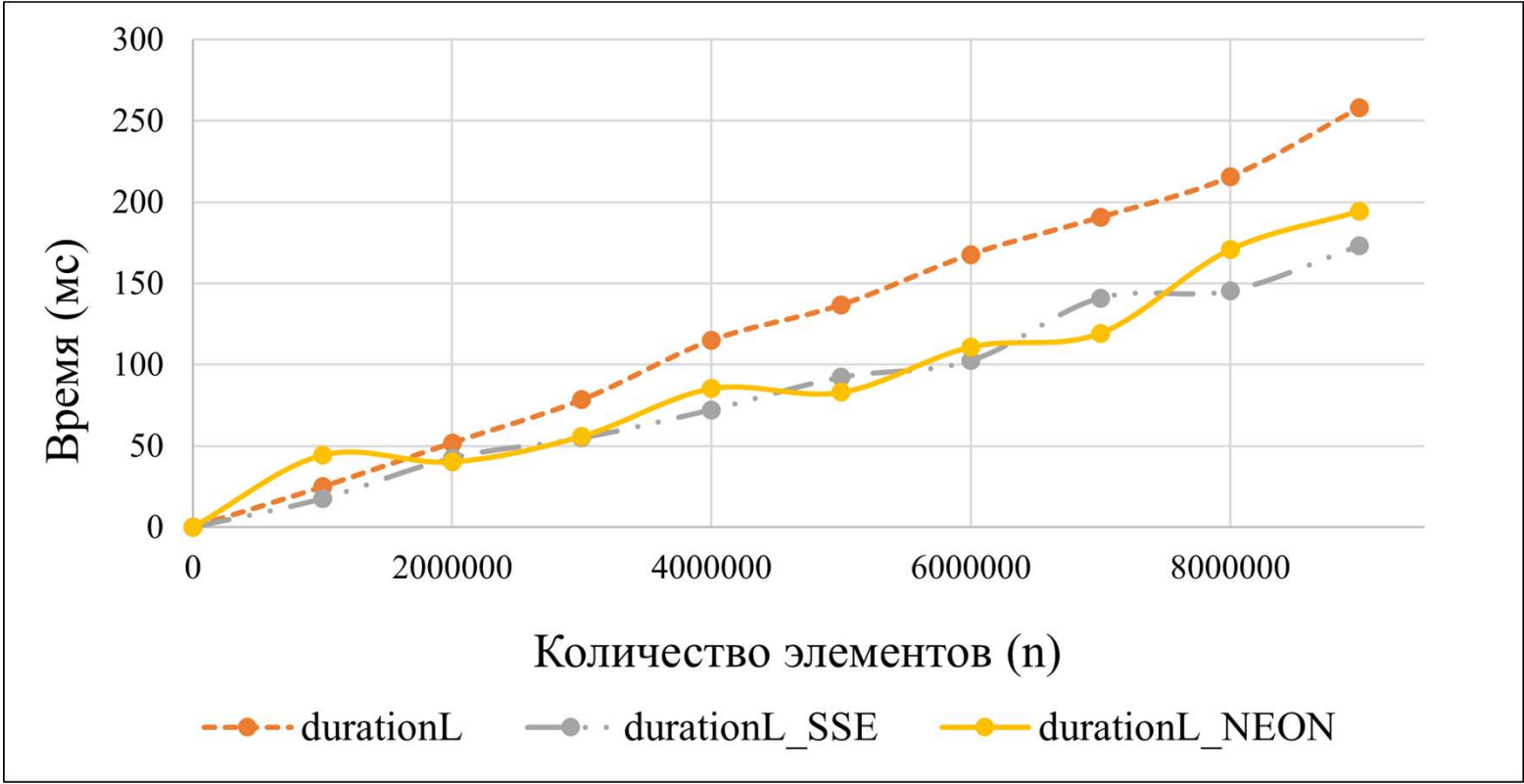
Рисунок 1 – График сравнений производительности алгоритма Левенштейна
