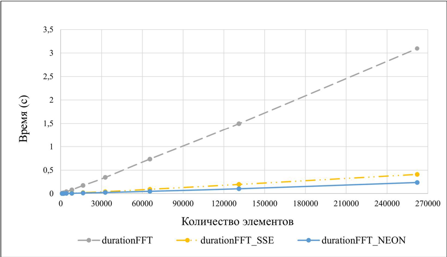
Рисунок 2 – График сравнений производительности алгоритма БПФ
